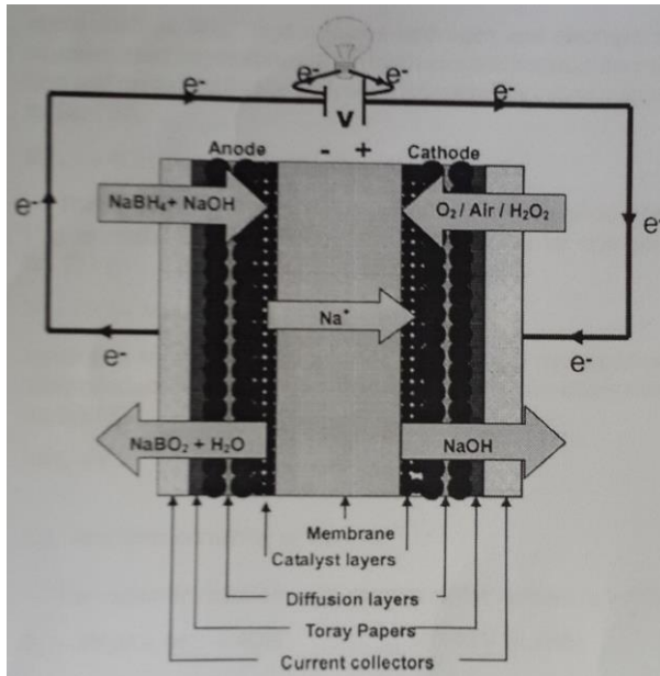
ნახაზი 11. ბორჰიდრიდის პირდაპირი დაჟანგვის საწვავი ელემენტის სქემატური დიაგრამა
